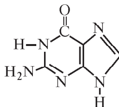
guanin (g)
