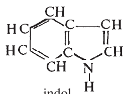
indol
