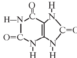
siydik kislotasi (2, 6, 7-trioksi purin)
