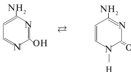
2-oksi-4-aminopirimidin (sitozin)
