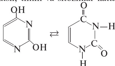
2. 4-dioksi pirimidin (uratsil)
