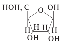
\beta -D-ribofuranaza
