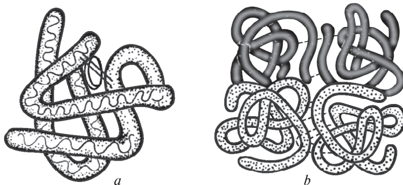
10-rasm. Oqsil molekulasining: a —uchlamchi, b —to'rtlamchi strukturasi.
