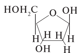
2-dezoksi- \beta -D-ribofuranaza
