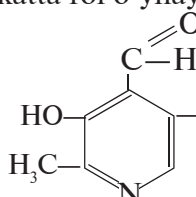
piridoksal
