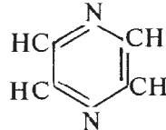
pirazin
