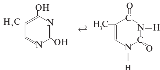
5-metil-2,4-dioksipirimidin (timin)
