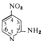
2-amino 4-nitro piridin
