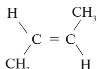
trans -2-buten
