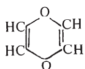
dioksin
