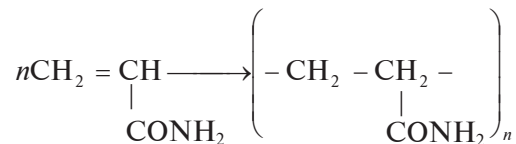
poliakrilamid
